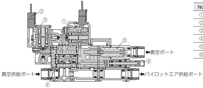
例).VXP-□□□-D24 (2ポート仕様単体タイプ 圧力センサ付)
