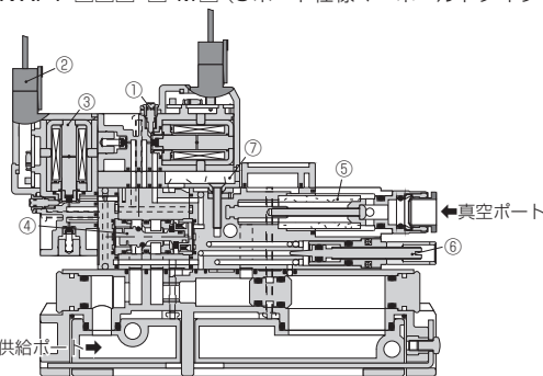
例).VXPT-□□□-□-D□-M□ (3ポート仕様マニホールドタイプ 圧力センサ付)
