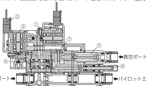
例).VXPT-□□□-D24 (3ポート仕様単体タイプ 圧力センサ付)
