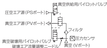
VXP-□□□-□-AO-(D)(ノーマルクローズタイプ)
