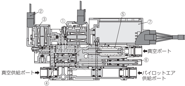
例).VXP□-□□□-□-M□ (2ポート仕様マニホールドタイプ 圧力センサ無し)
