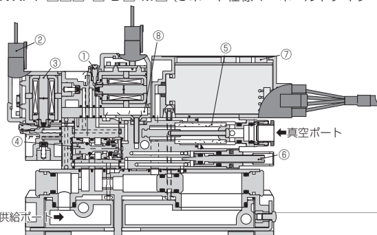
例).VXPT-□□□-□-D□-M□ (3ポート仕様マニホールドタイプ 圧力センサ付)
