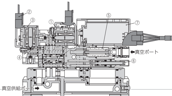
例).VXP□-□□□-□-D□-M□ (2ポート仕様マニホールドタイプ 圧力センサ付)
